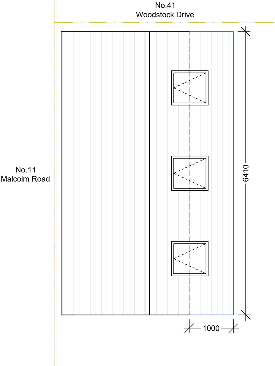
○ R o o f P l a n 1 : 5 0
