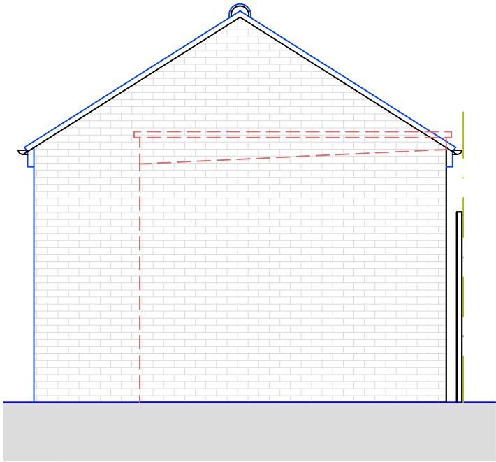
○ R e a r E l e v a t i o n 1 : 5 0
