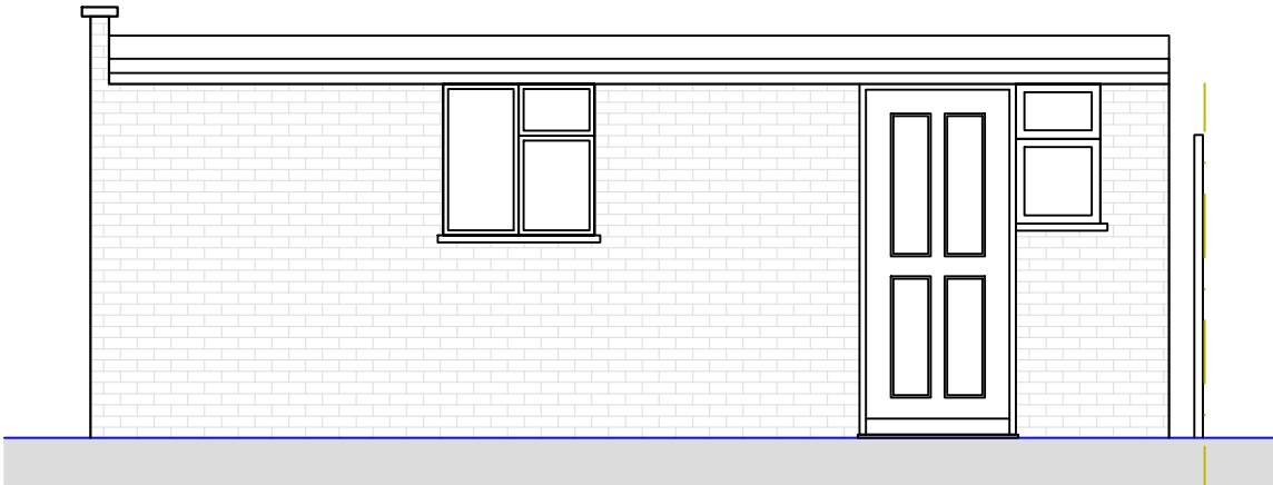
Side Elevation 2 1:50
