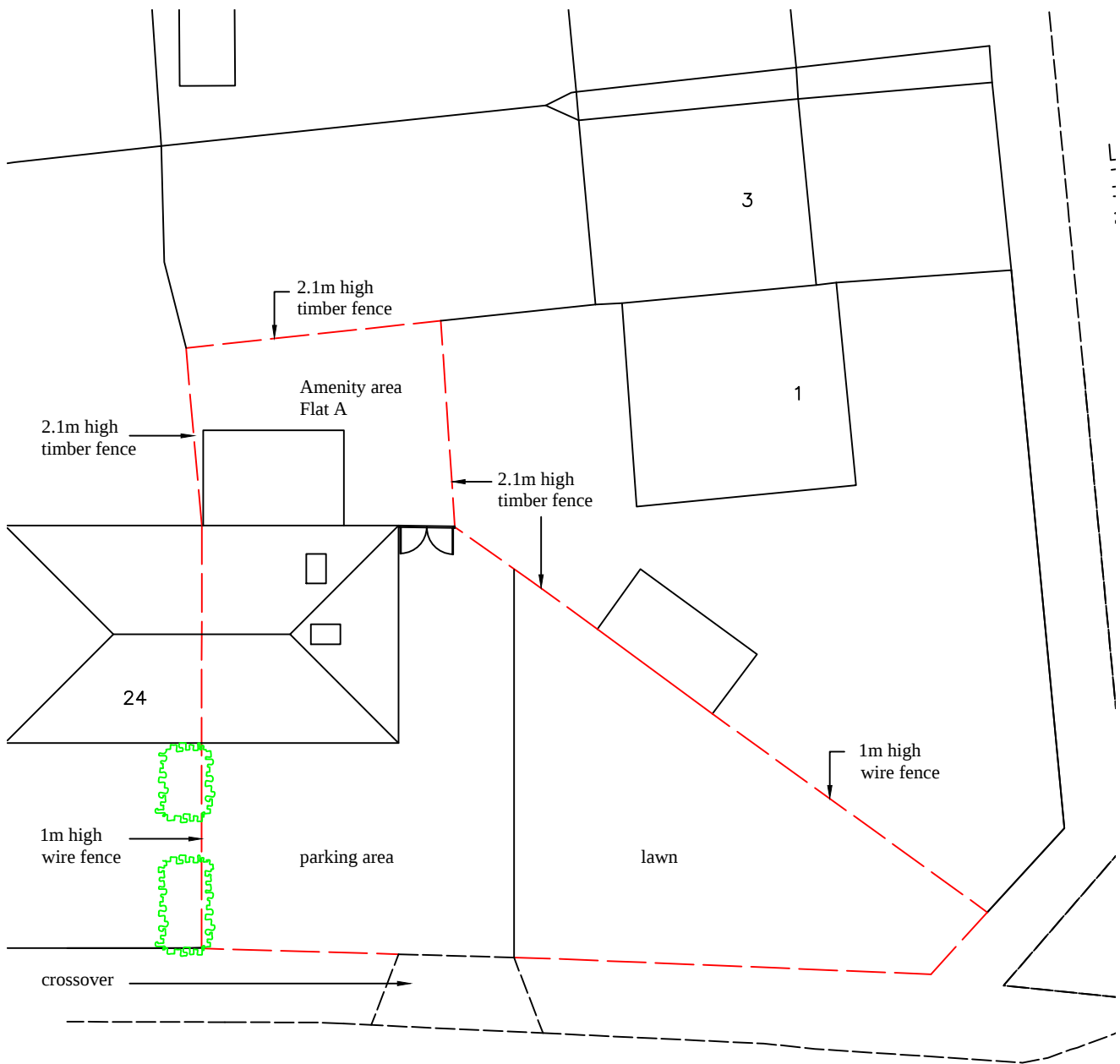
Site Plan 1:200
