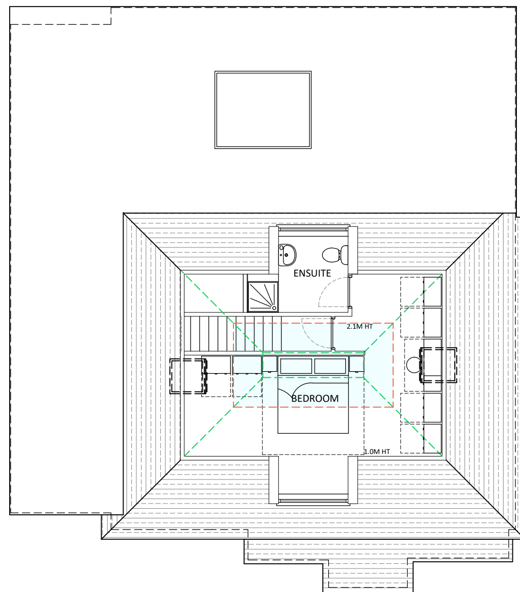
LOFT PLAN
