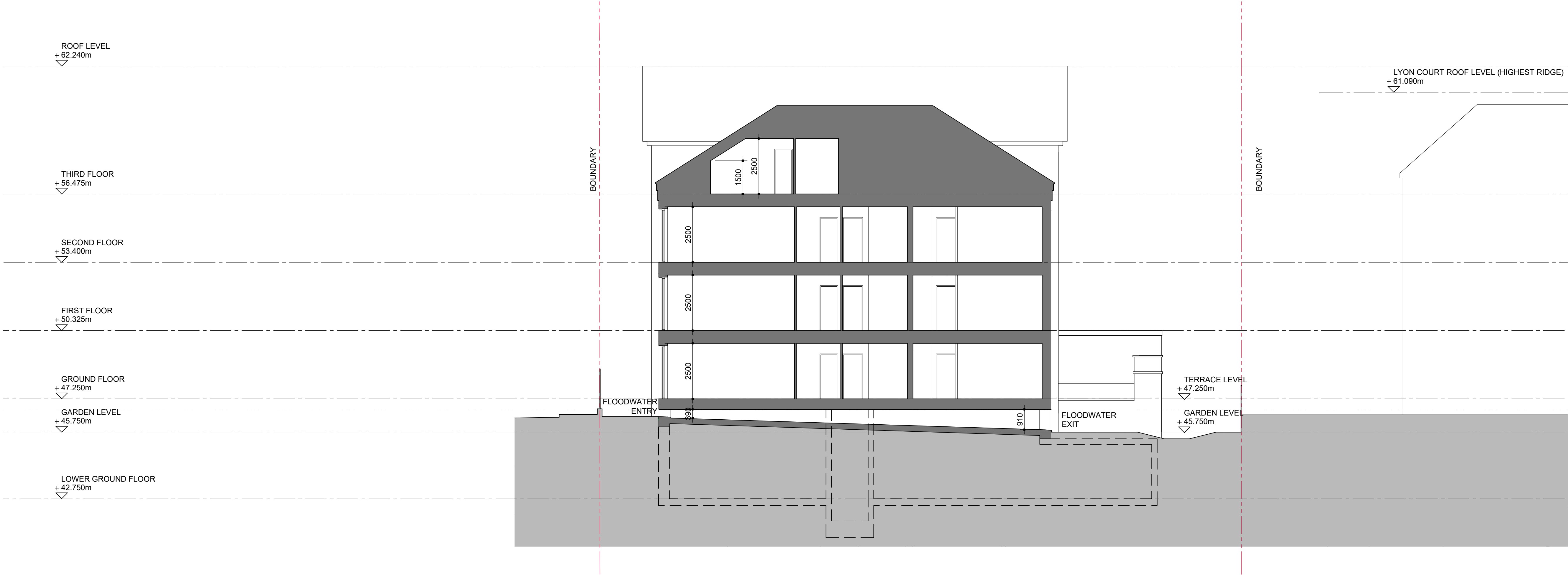
SECTION B-B 1:100 @ A1
