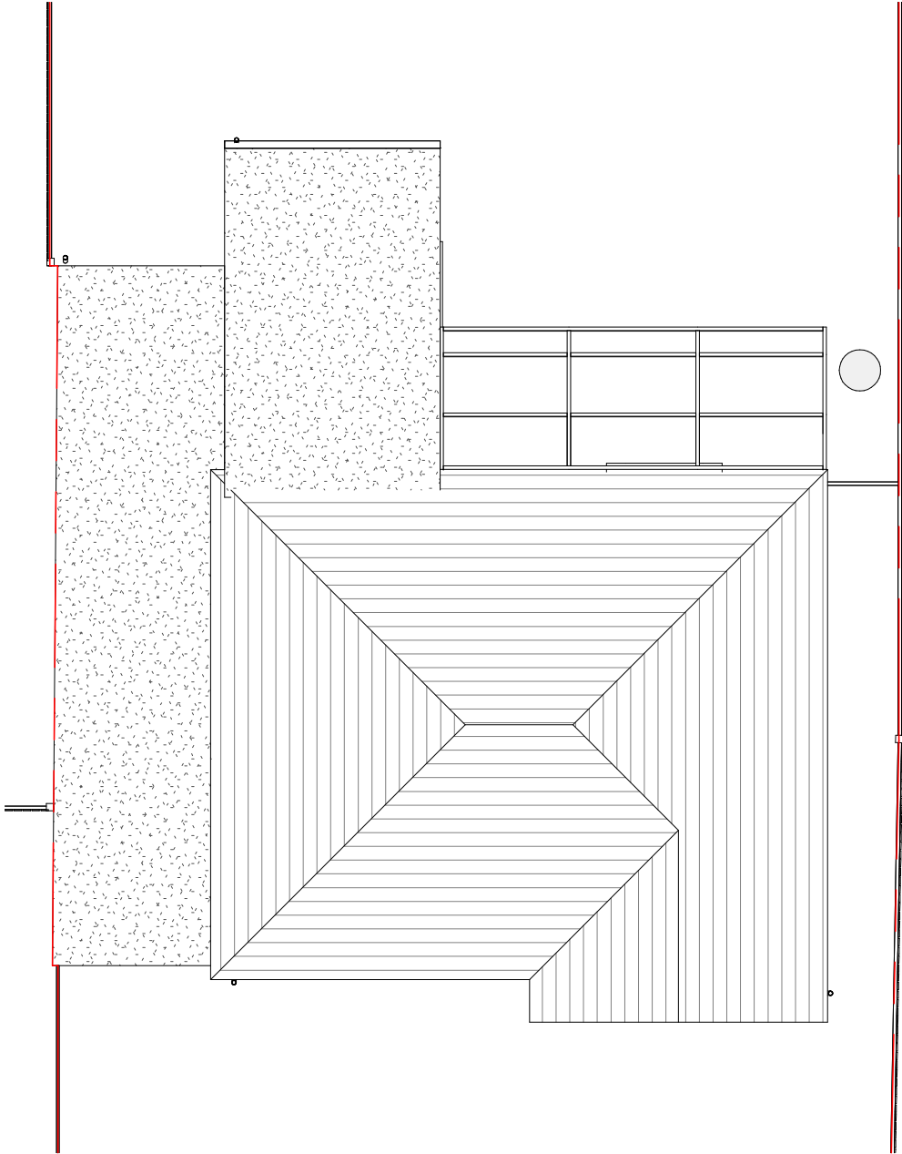
ROOF PLAN 1 : 100
