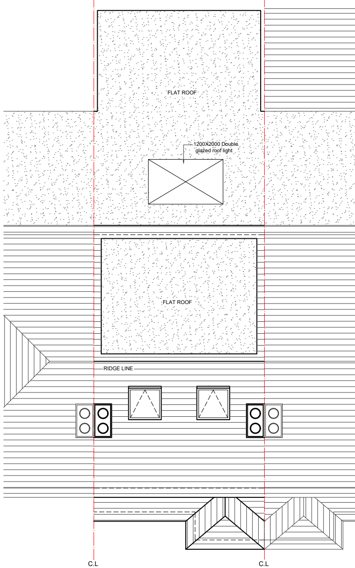
03 - LOFT PLAN
