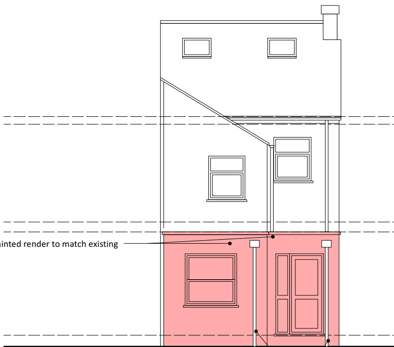
2 SOUTH Scale: 1:100
