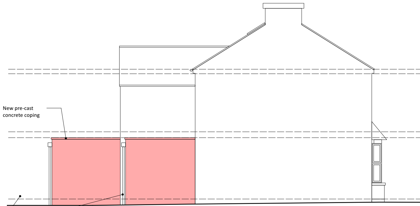
3 EAST Scale: 1:100
