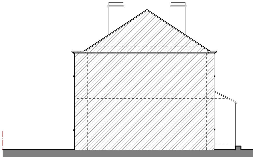
4 NORTH Scale: 1:100
