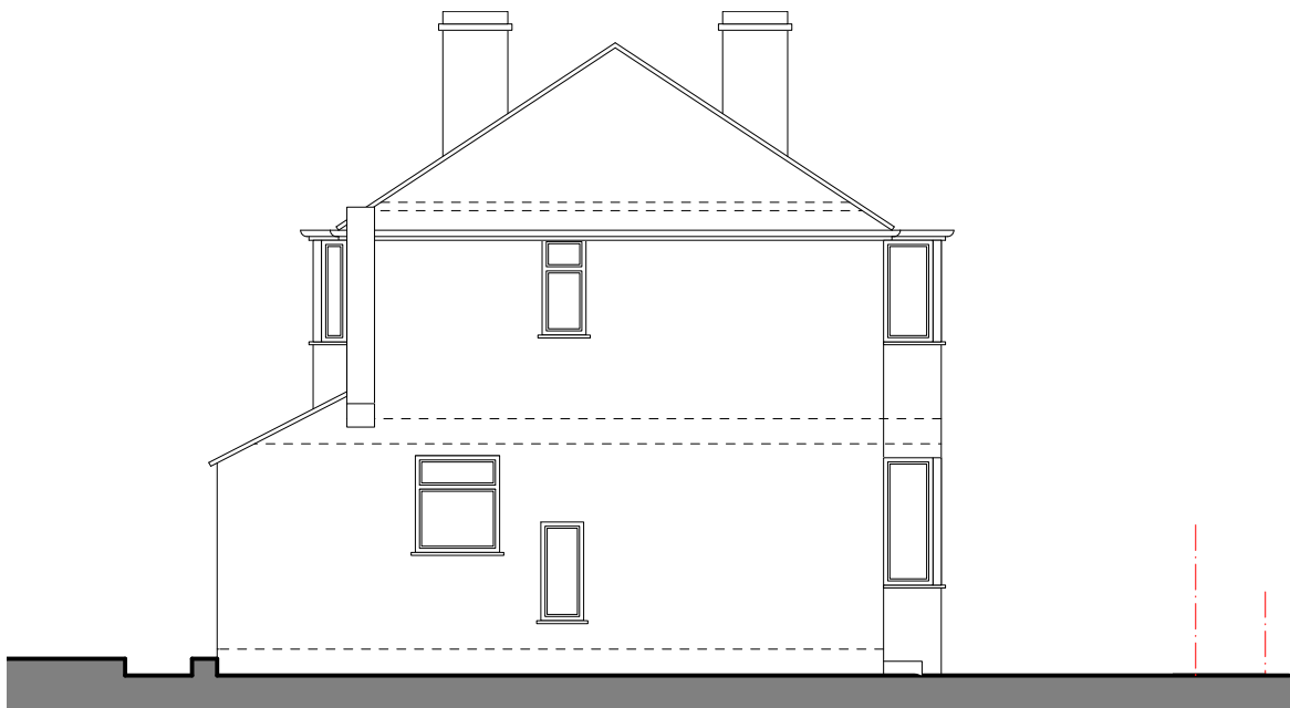
3 SOUTH Scale: 1:100
