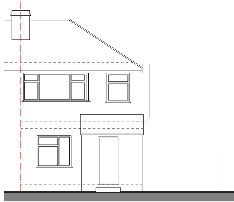
2 WEST Scale: 1:100
