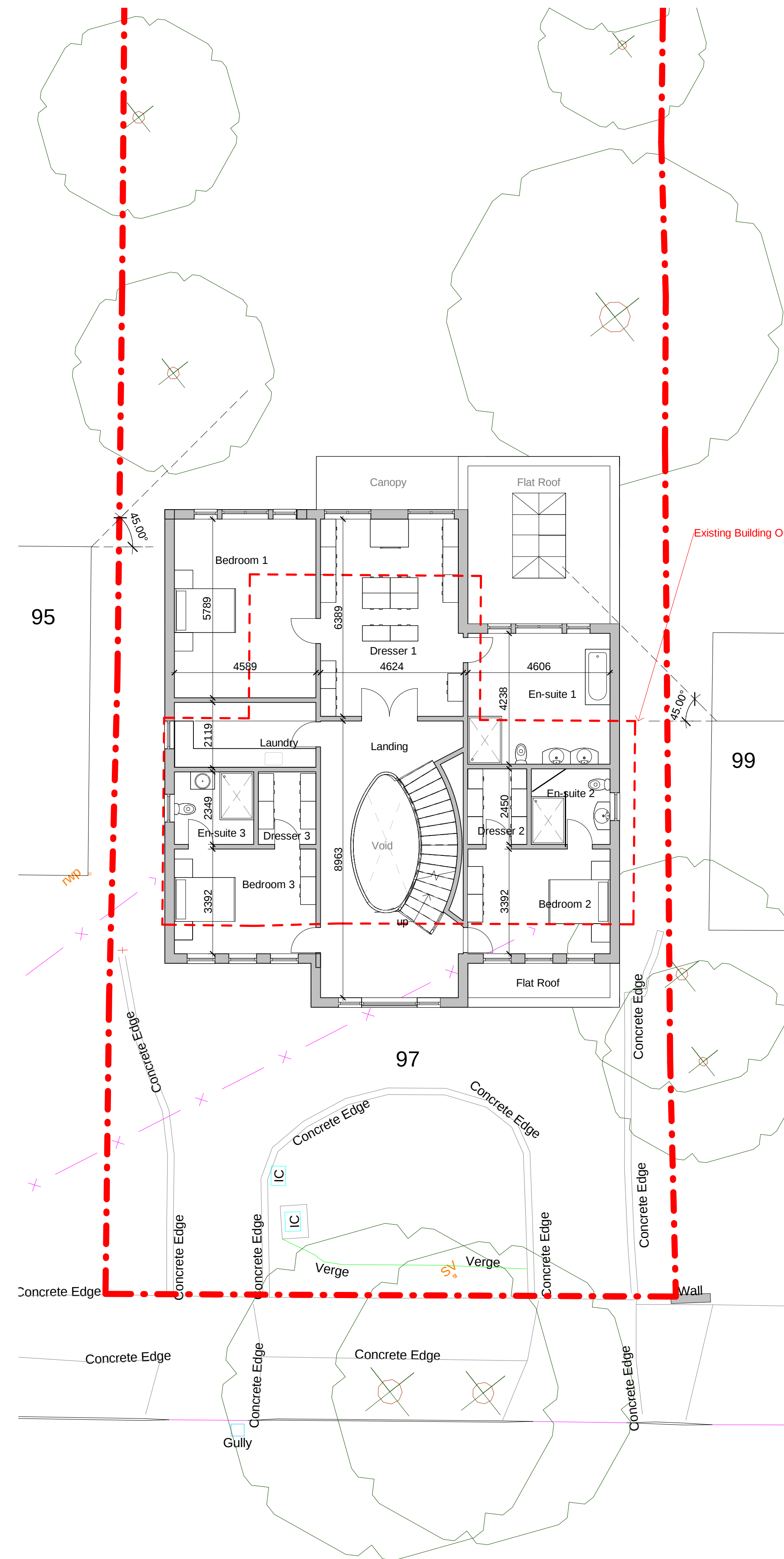
2 02.First Floor 1 : 100
