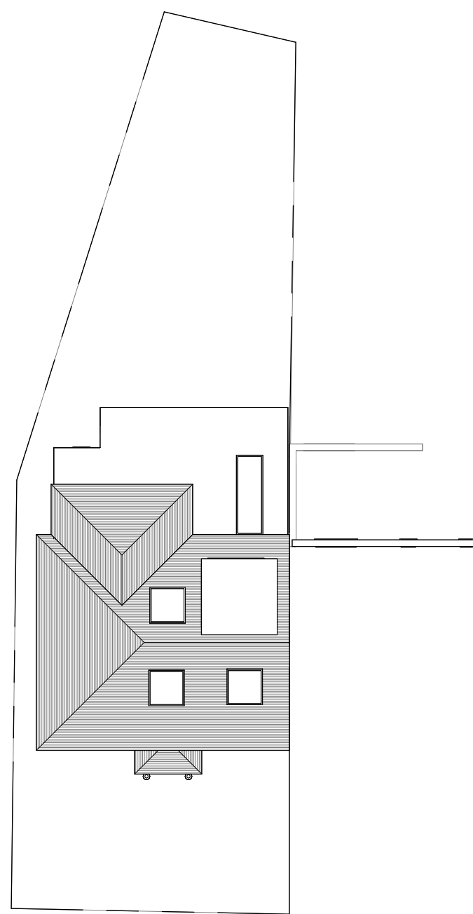
1 Site Plan 1:200
