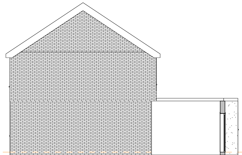
7 Right Elevation 1 : 100
