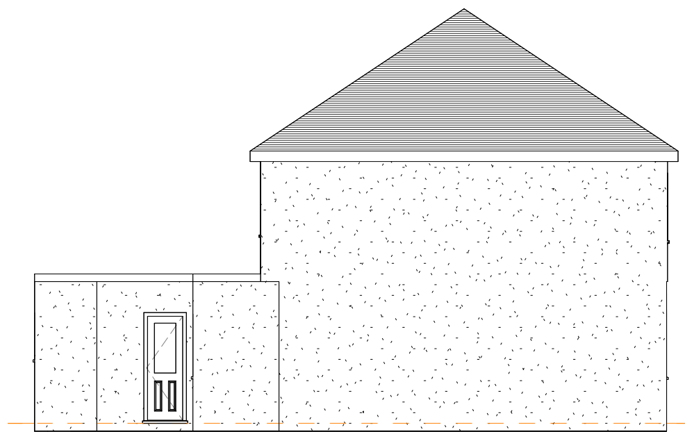
5 Left Elevation 1 : 100
