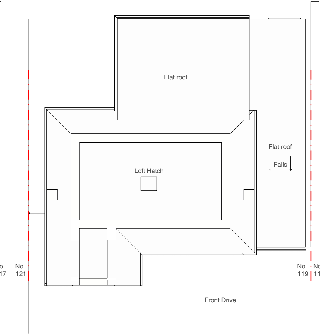
Loft Plan
