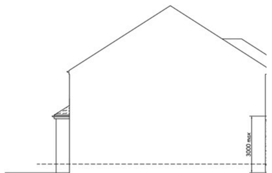
FLANK ELEVATION
