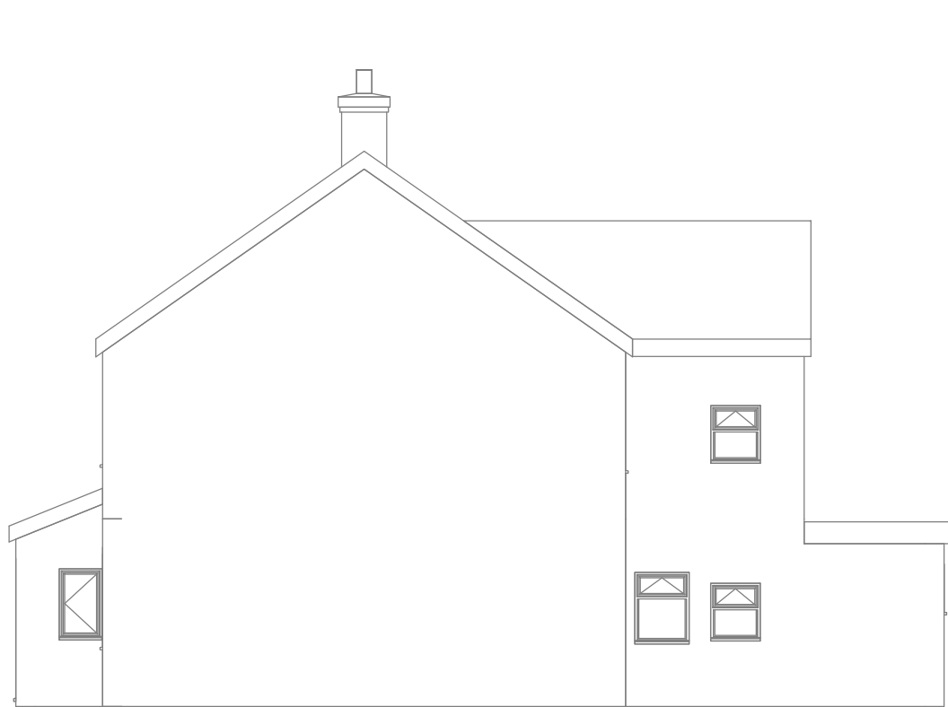
Right Side 1 : 100
