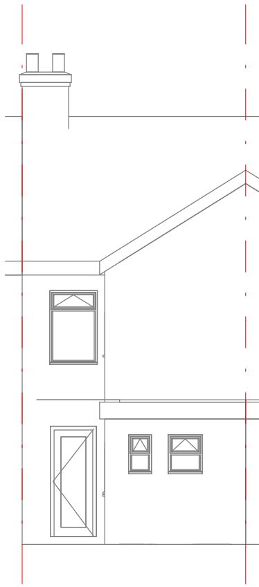
Rear 1 : 100
