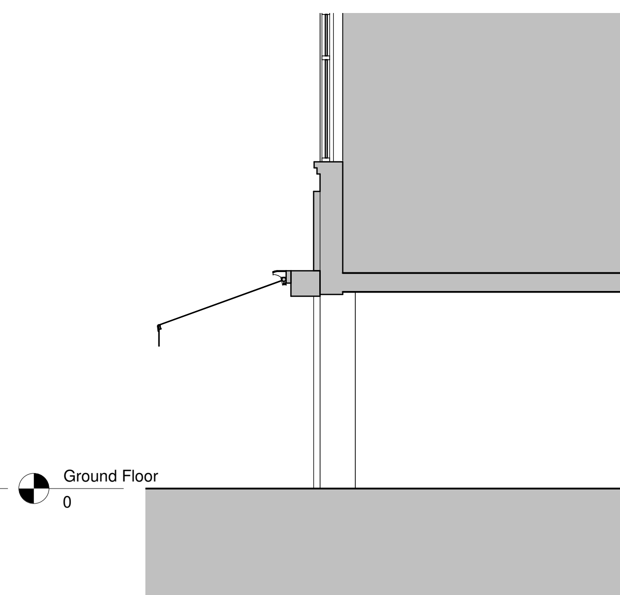
Section AA Open Canopy 1 : 50
