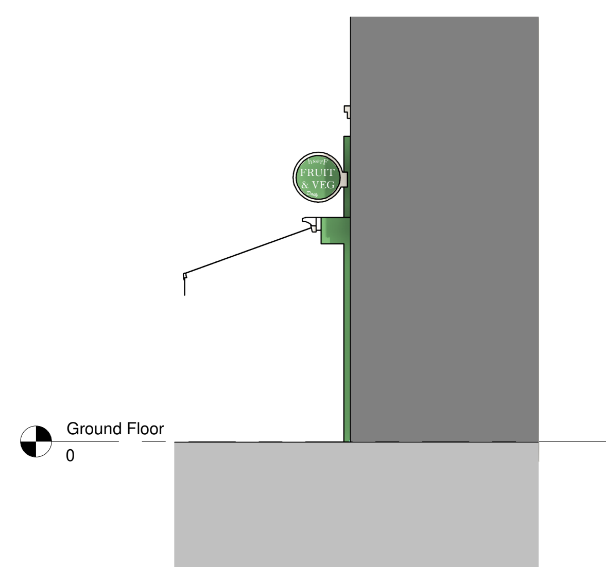
Right Elevation 1 : 50
