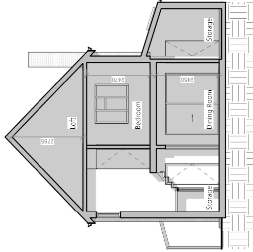
② Existing section1 1 : 100
