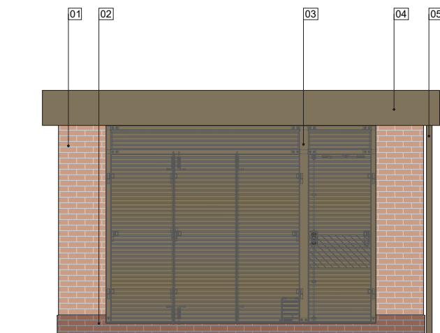
Elevation B-B'
