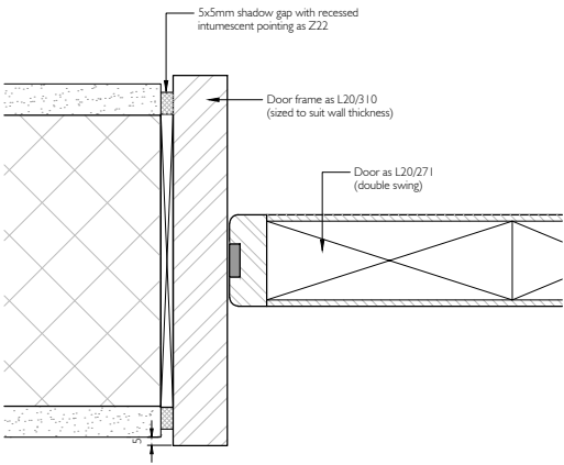
1 DOOR TYPE 5 - JAMB DETAIL
