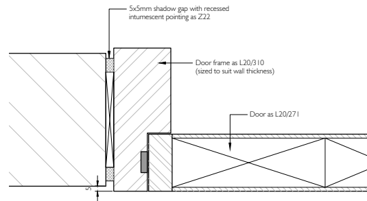
9 DOOR TYPE 11 - JAMB DETAIL
