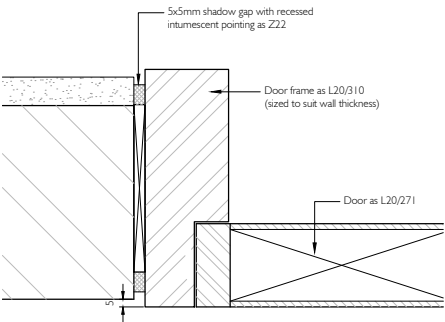
7 DOOR TYPE 8 & 10 - JAMB DETAIL
