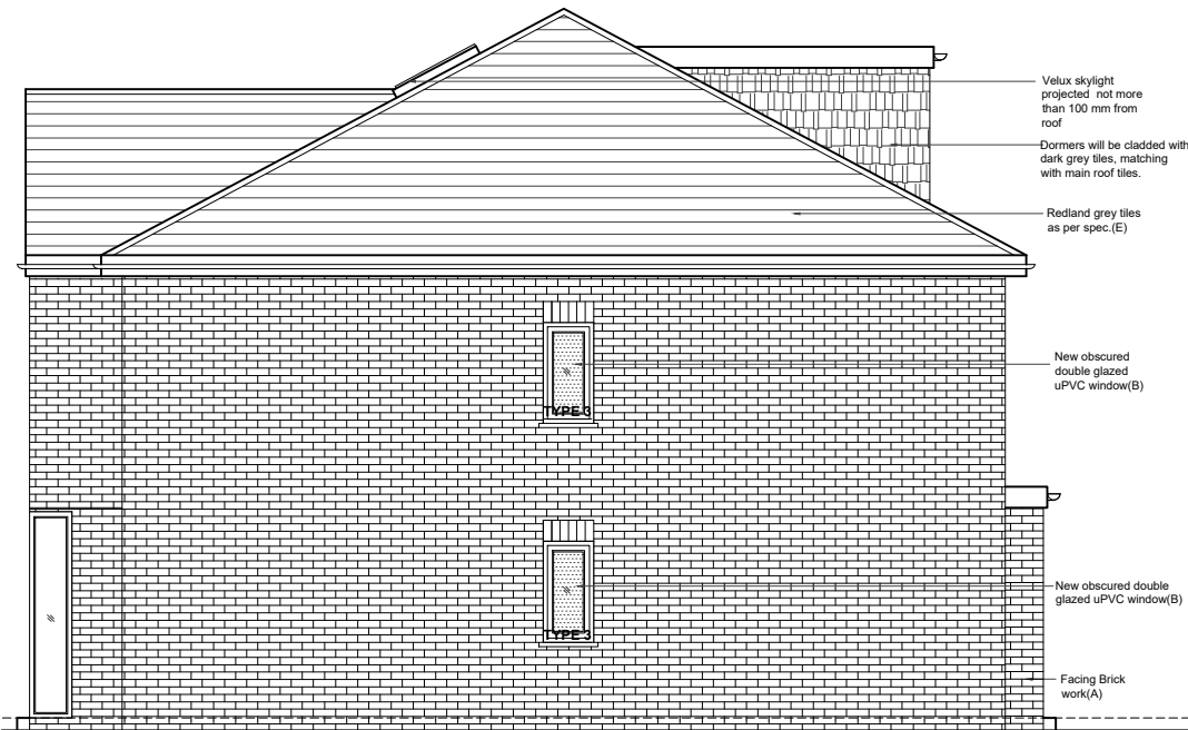
01 -FRONT ELEVATION
