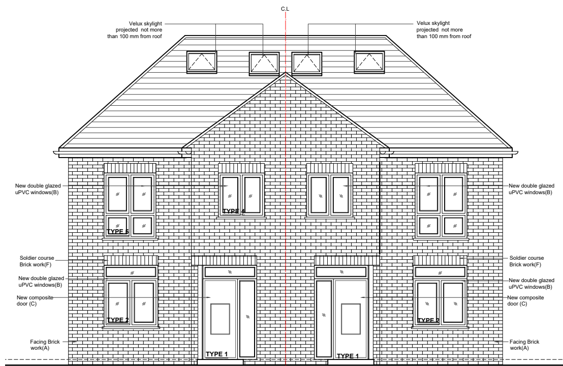
01 -FRONT ELEVATION
