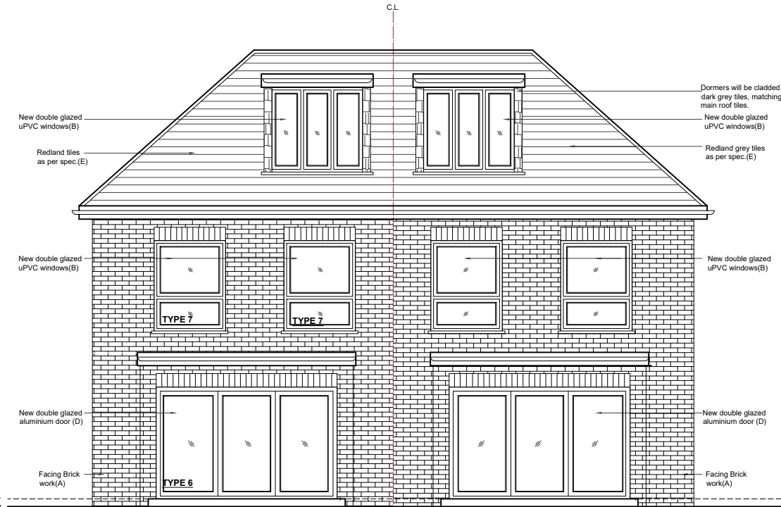
02 -REAR ELEVATION
