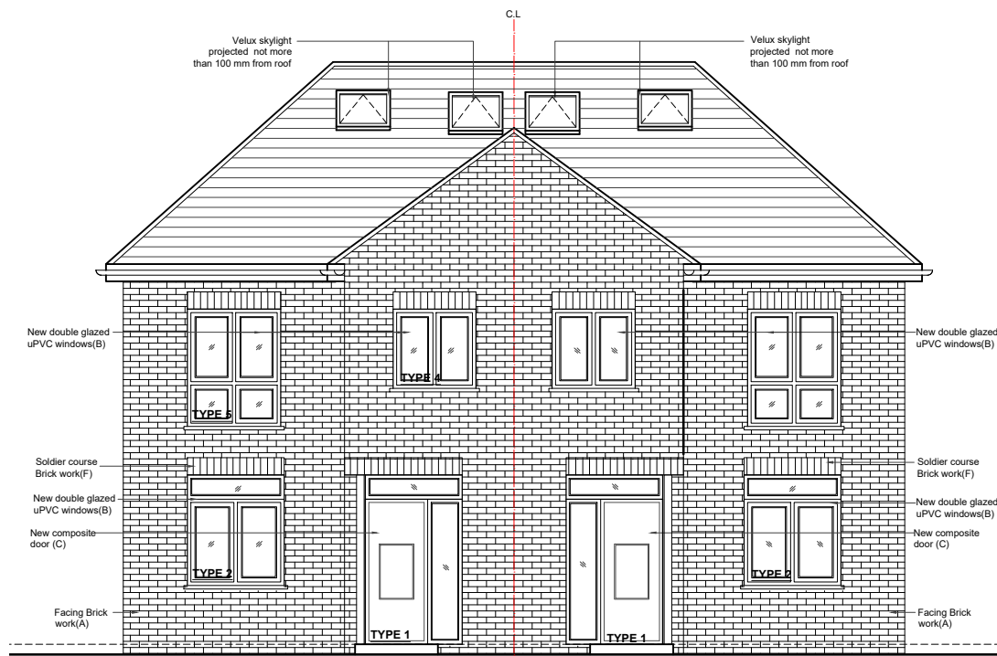
01 -FRONT ELEVATION
