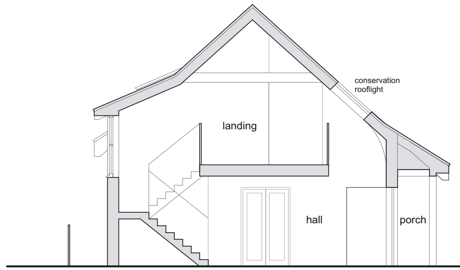
06 Section DD 1:100@A3; 1:50@A1
