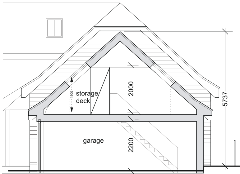
04 Section BB 1:100@A3; 1:50@A1
