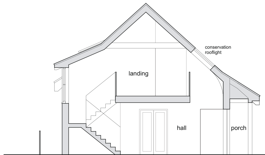
06 16 Section DD 1:100@A3; 1:50@A1
