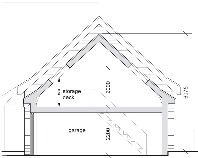
04 16 Section BB 1:100@A3; 1:50@A1
