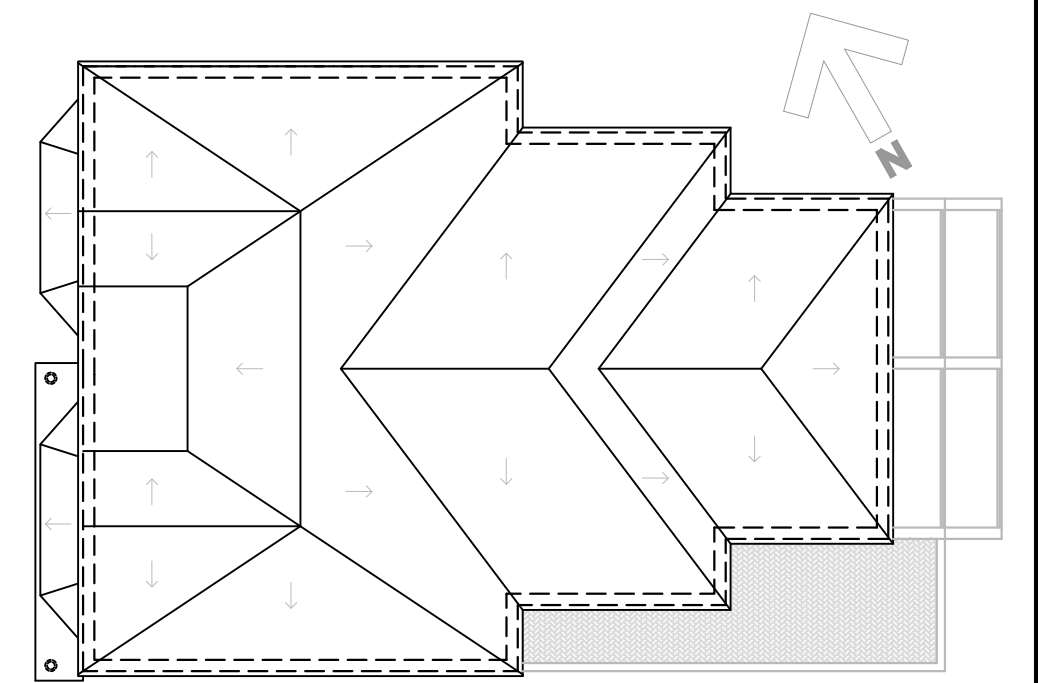
SCALE - 1:200
